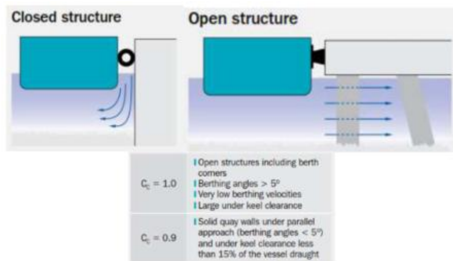
Gambar 3.7 Penentuan koefisien C_c
