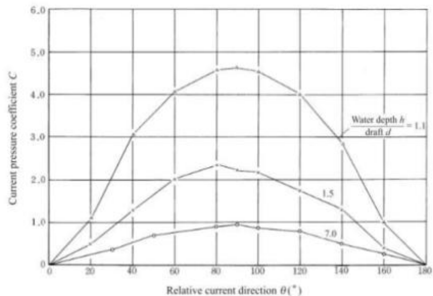
Gambar 3.9 Koefisien tekanan arus
