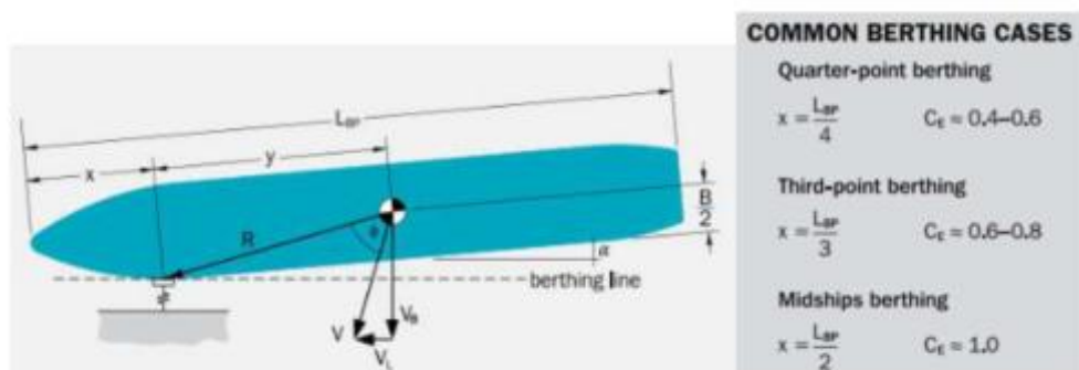
Gambar 3.6 Penentuan Koefisien CE
