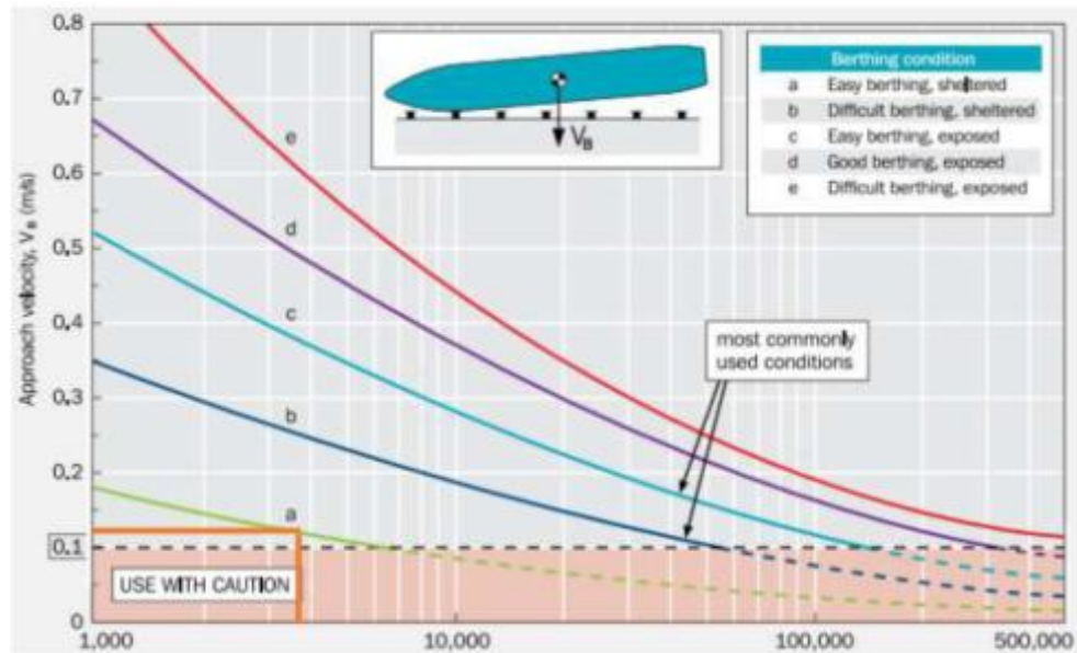
Gambar 3.4 Grafik kecepatan kapal bertambat
