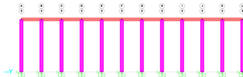
Gambar 0.3 Pemodelan Spring Dermaga dengan SAP2000
