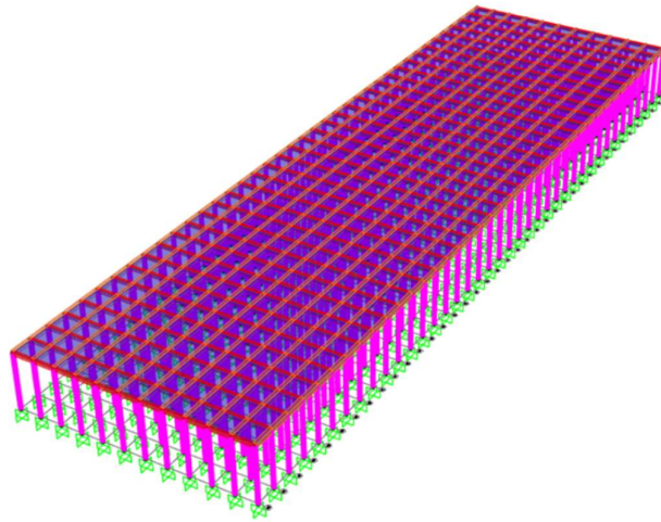
Gambar 0.2 Tampak Perspektif Pemodelan Dermaga dengan SAP2000
