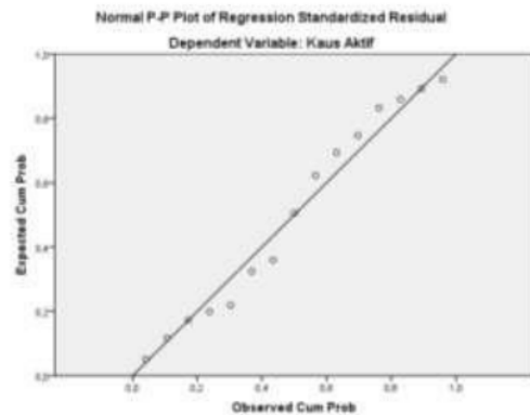
Gambar 7. Normal Plot Kasus Aktif
