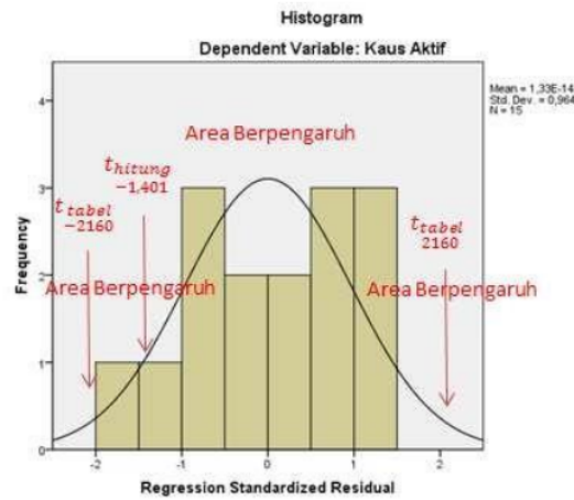
Gambar 6. Kurva Hasil Uji Regresi Sederhana
