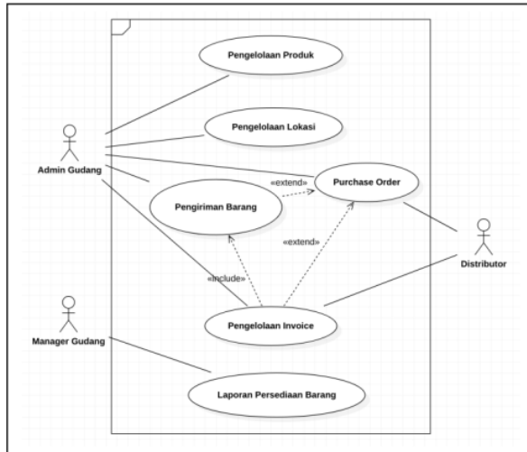
Gambar 4. Use case Diagram Sistem Informasi Distribusi Barang
