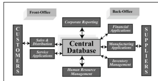
Gambar 3. Konsep ERP
