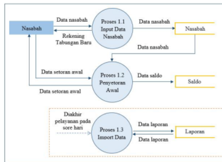
Gambar 5. Data Flow Diagram (DFD) Level 1 Proses 1.0 Sistem Yang Diusulkan
