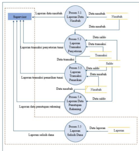
Gambar 6. Data Flow Diagram (DFD) Level 1 Proses 5.0 Sistem Yang Diusulkan
