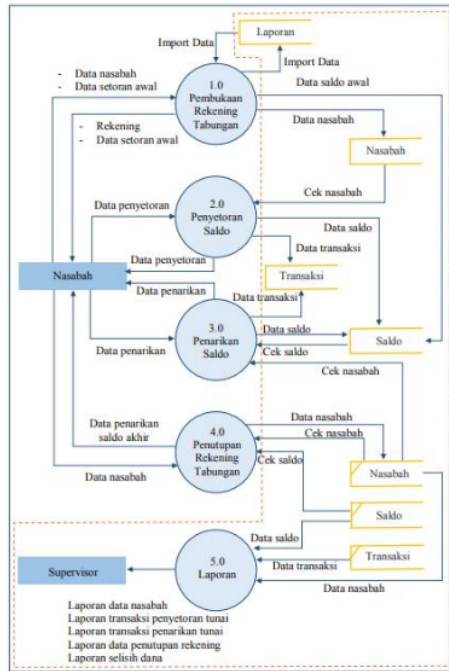
Gambar 4. Data Flow Diagram (DFD) Level 0 Sistem Yang Diusulkan
