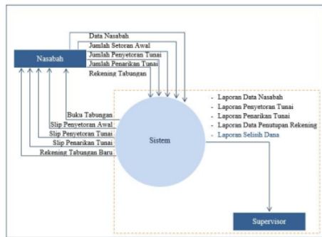
Gambar 3. Diagram Konteks Sistem Yang Diusulkan
