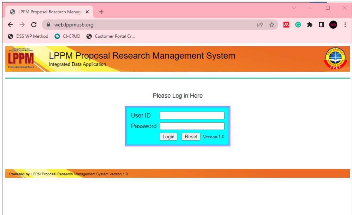
Gambar 2. Halaman Login
