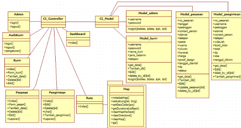
Gambar 3. Class Diagram TSP menggunakan Algoritma Genetika
