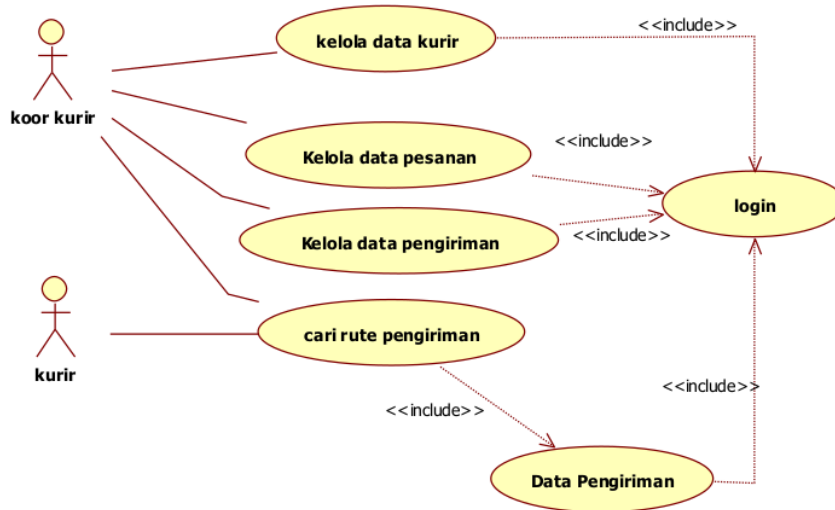
Gambar 2. Use Case Diagram TSP menggunakan Algoritma Genetika
