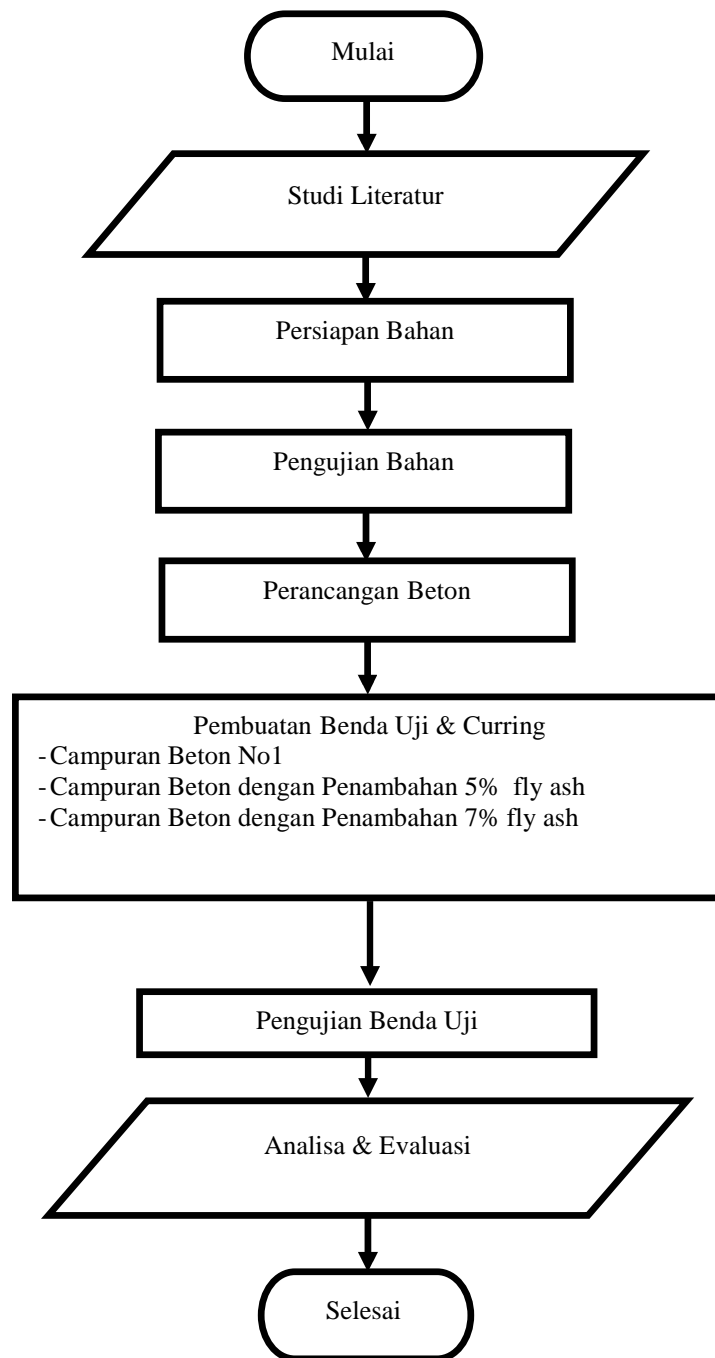
Gambar 3.1 Metodologi Penelitian
